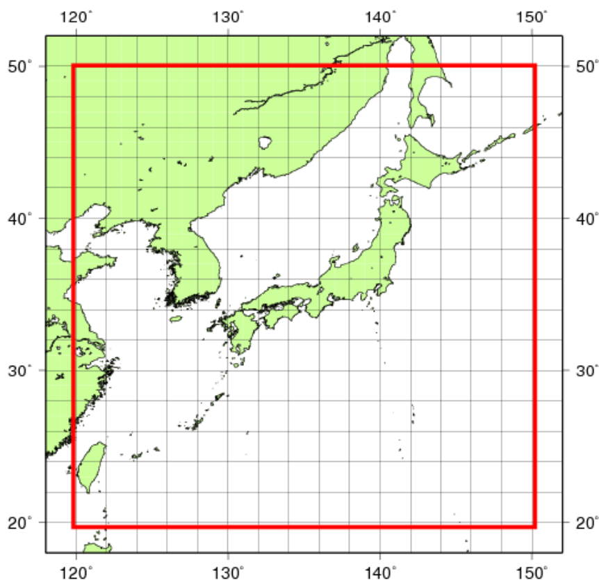
図 1 JRA-3Q プロダクト (日本域セット) の領域 赤線の範囲内が対象となる領域
