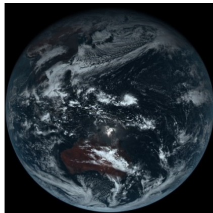
平成 26 年 12 月 18 日午前 11 時 40 分（日本時間）、 ひまわり 8 号によって撮影された画像 （可視 3 バンド合成カラー画像）
